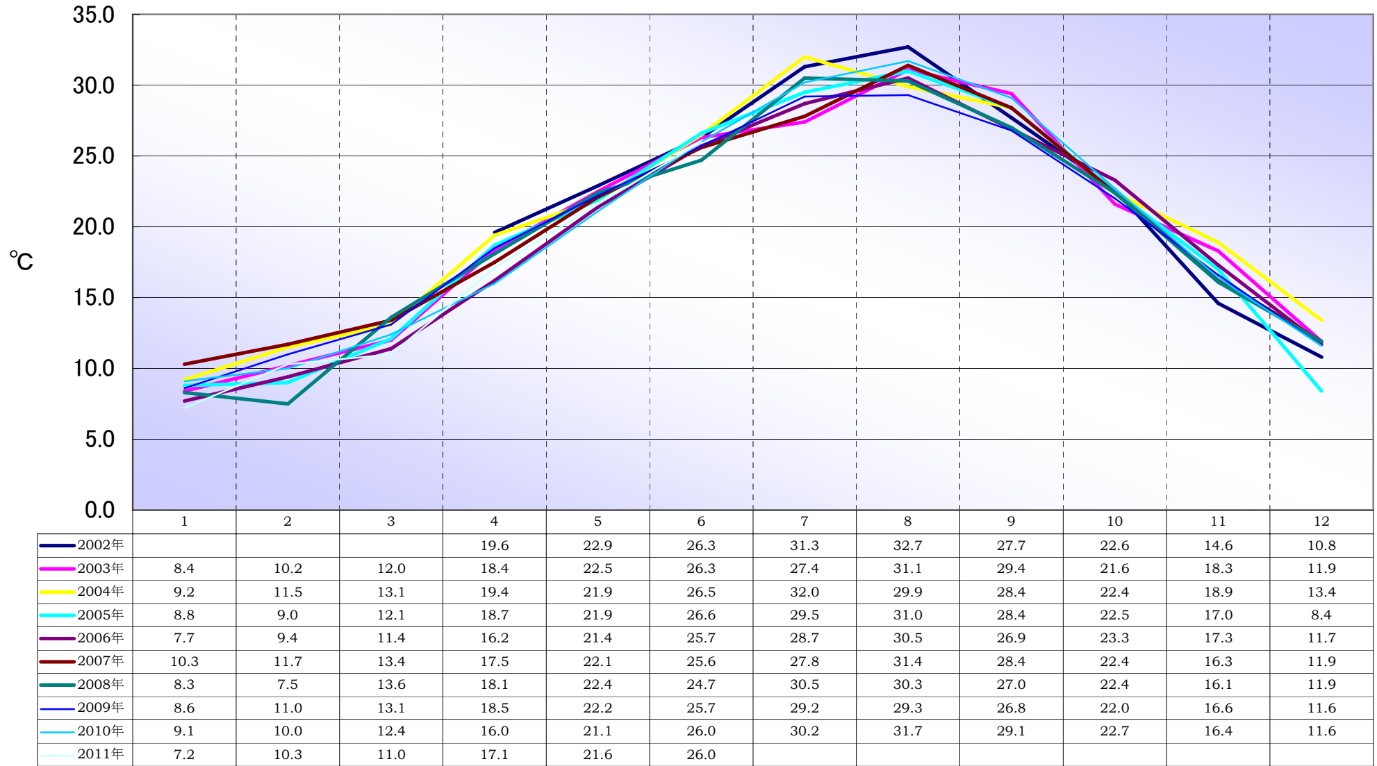
各年の日最高気温平均値のグラフ ～三重県鈴鹿市磯山～
