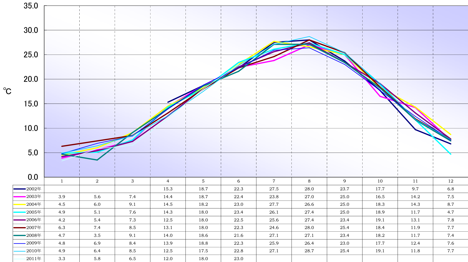
各年の月平均気温のグラフ ~三重県鈴鹿市磯山~
